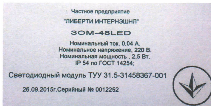
Фото 3. Маркировка заградительного огня «ЗОМ-48LED».
