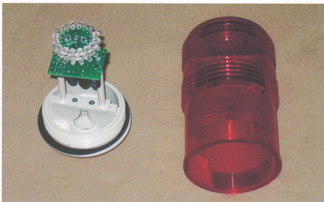
Фото 2. Внешний вид заградительного огня «ЗОМ-48LED» без поликарбонатной части, пропускающей свет.
