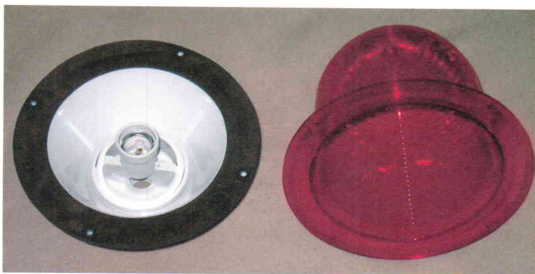
Фото 2. Внешний вид заградительного огня «ЗОМ-150Вт» без поликарбонатной части, пропускающей свет.
